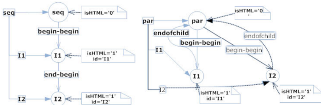
Figure 17: La représentation d'ordonnancement de (a) conteneur "seq" et (b) conteneur "par"
