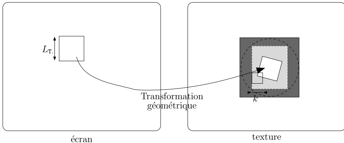
FIG. 7.15 – Zone de texture potentiellement accédée lors du rendu d’une tuile.
