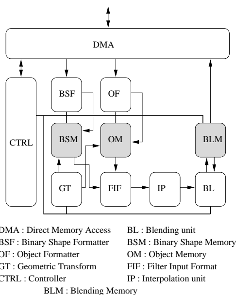
FIG. 9.7 – Diagramme en blocs du compositeur d'objet vidéo. Les mémoires internes apparaissent en grisées.
