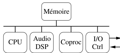
FIG. 2.1 – Architecture typique d'un système pour portable.
